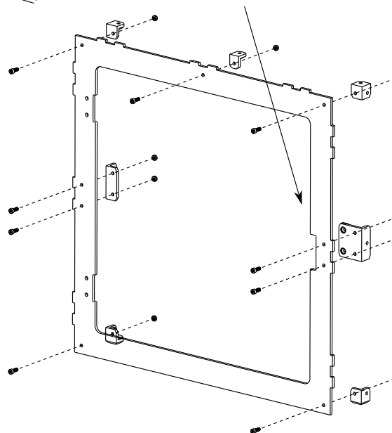
Instalace dveří: levá varianta Left Hand Door Installation
