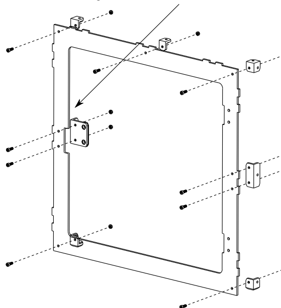
Instalace dveří: pravá varianta Right Hand Door Installation
